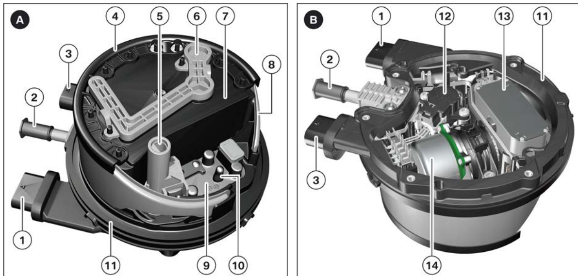
SCR 3, tank flange module
